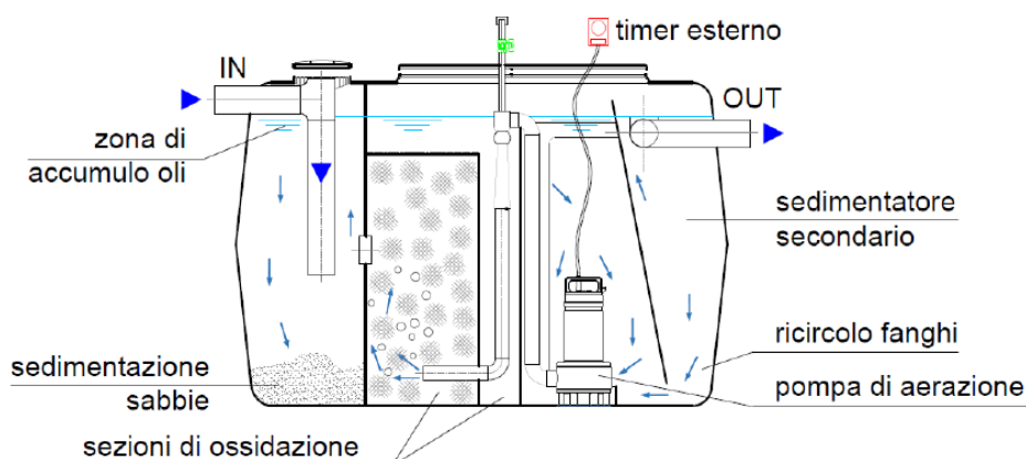
Figura n. 10 - Particolare costruttivo (sezione) del sistema di trattamento fisico-biologico delle acque di lavaggio
