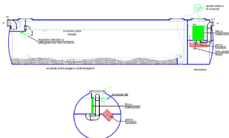
Figura 12 - Particolari costruttivi e sezione dell'impianto di trattamento delle acque di prima pioggia
